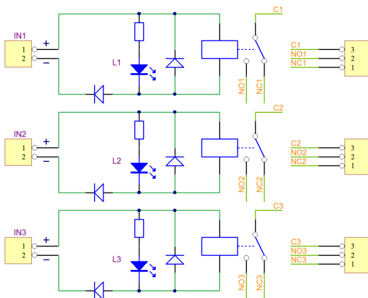
Rys. 2. Schemat elektryczny.
